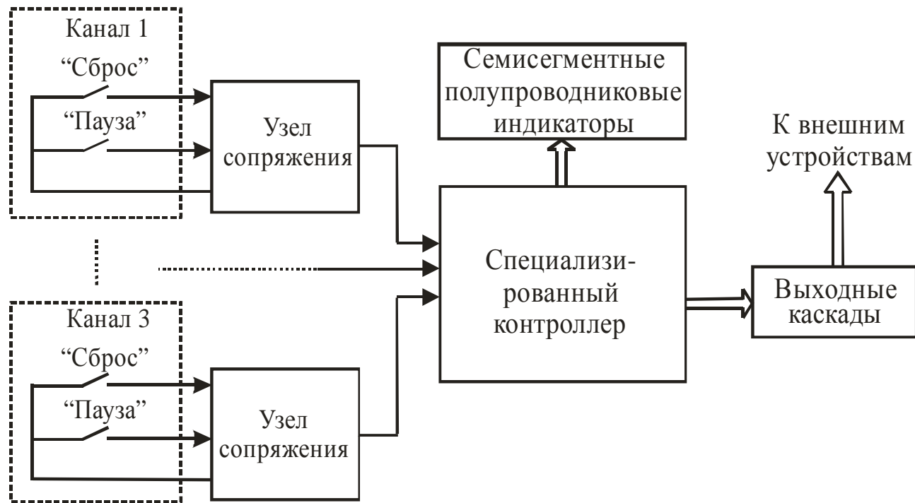
Рисунок 3.1 – Обобщенная функциональная схема прибора
