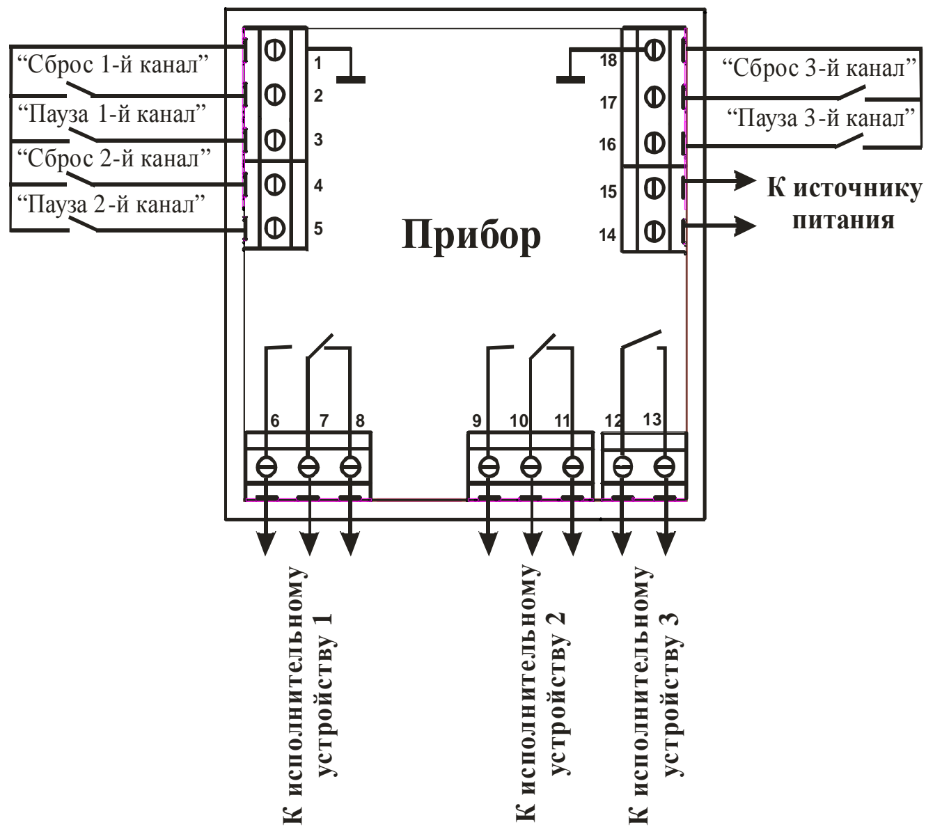
Рисунок 8.1 – Схема подключения источника питания и внешних устройств
