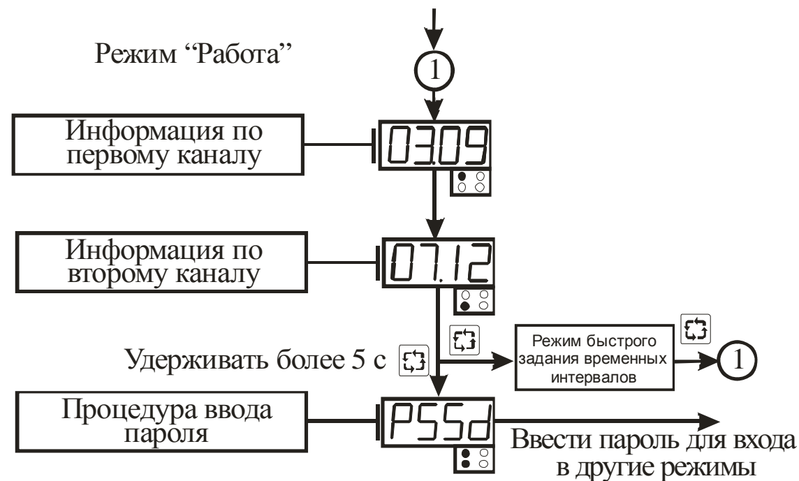
Рисунок 3.5 – Алгоритм работы прибора в режиме "Работа"
