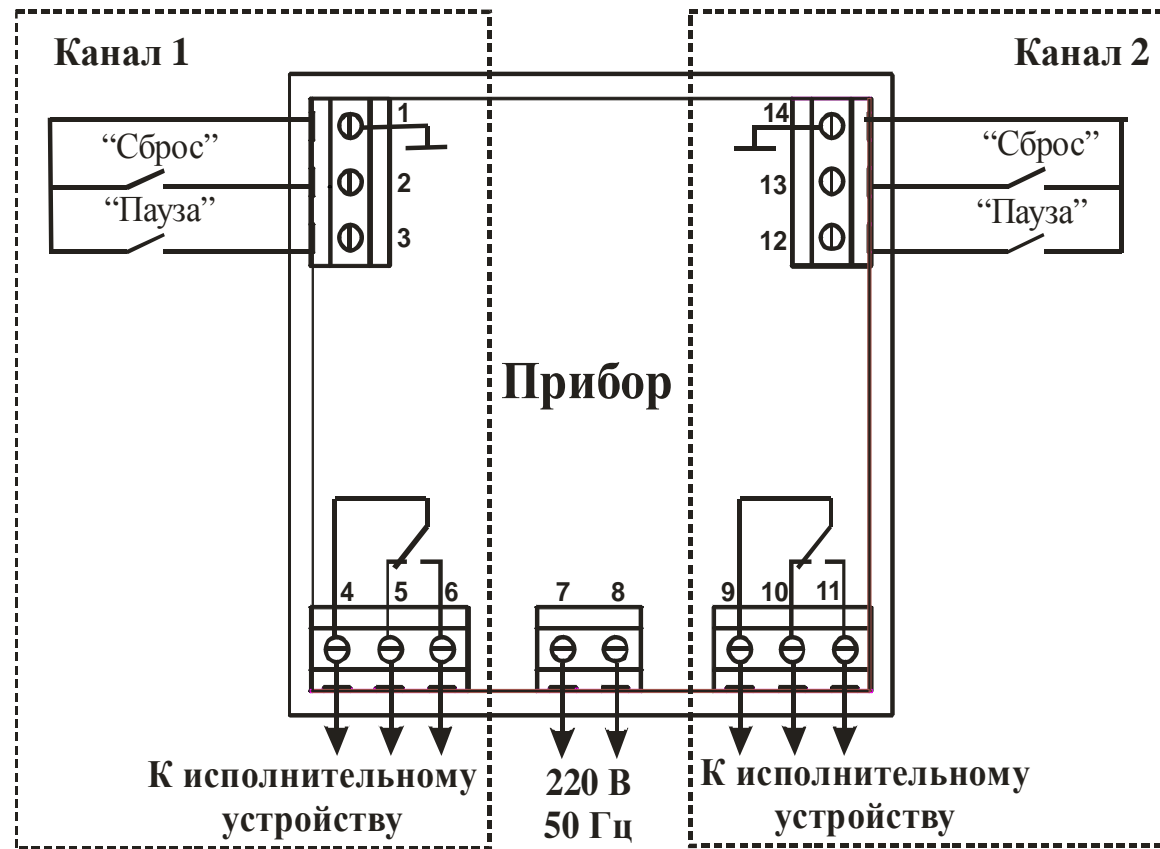
Рисунок 8.1 – Схема подключения источника питания и внешних устройств
