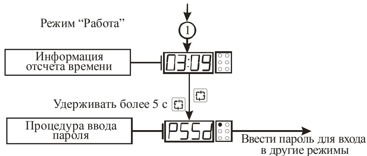
Рисунок 3.5 – Алгоритм работы прибора в режиме "Работа"
