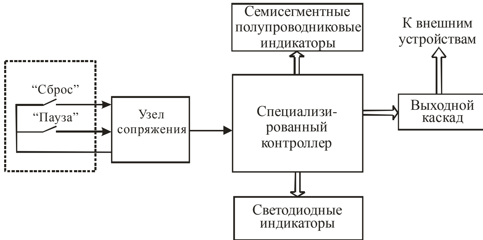
Рисунок 3.1 – Обобщенная функциональная схема прибора
