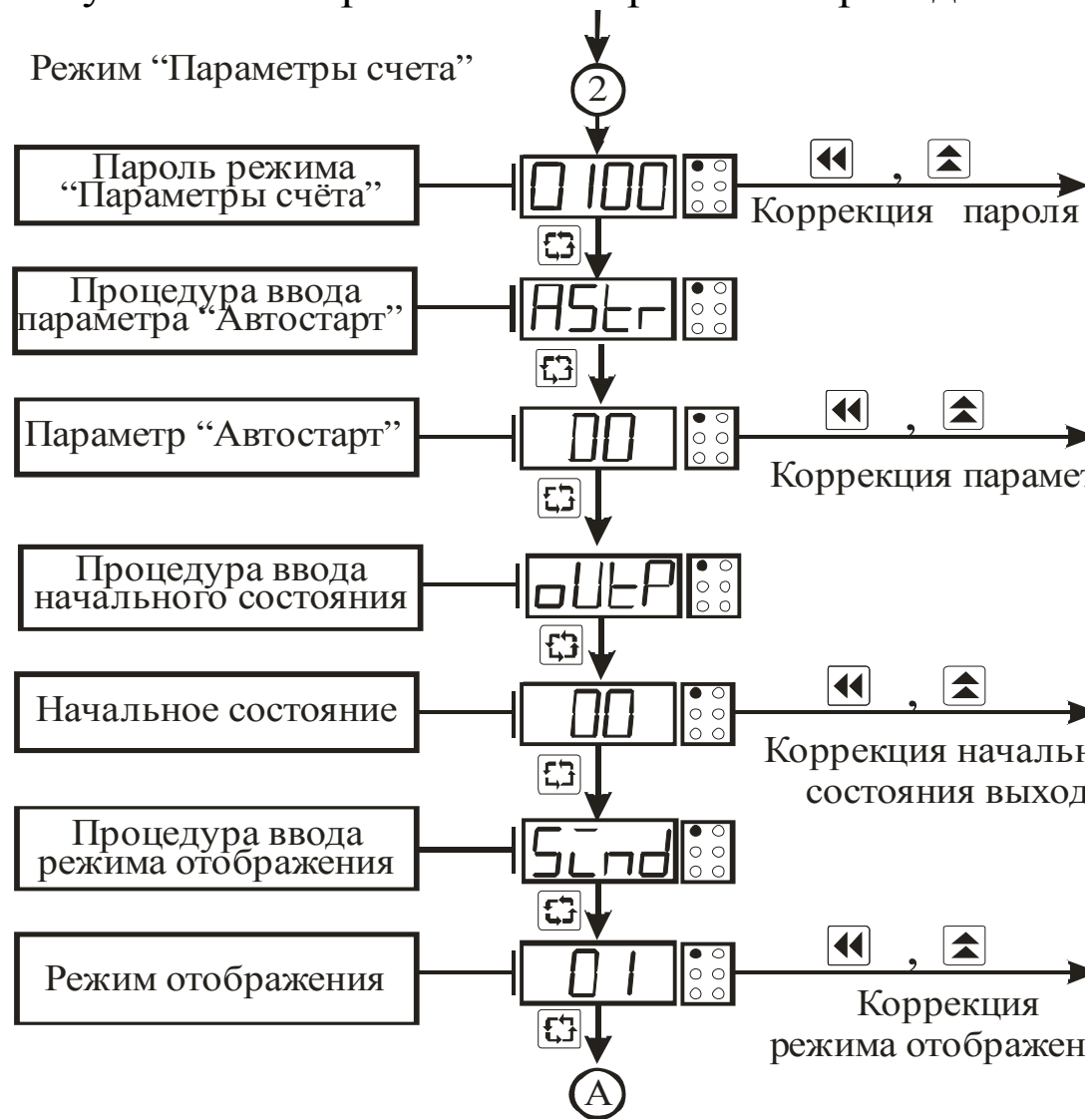
Рисунок 3.6 – Схема алгоритма работы в режиме “Параметры счёта”
