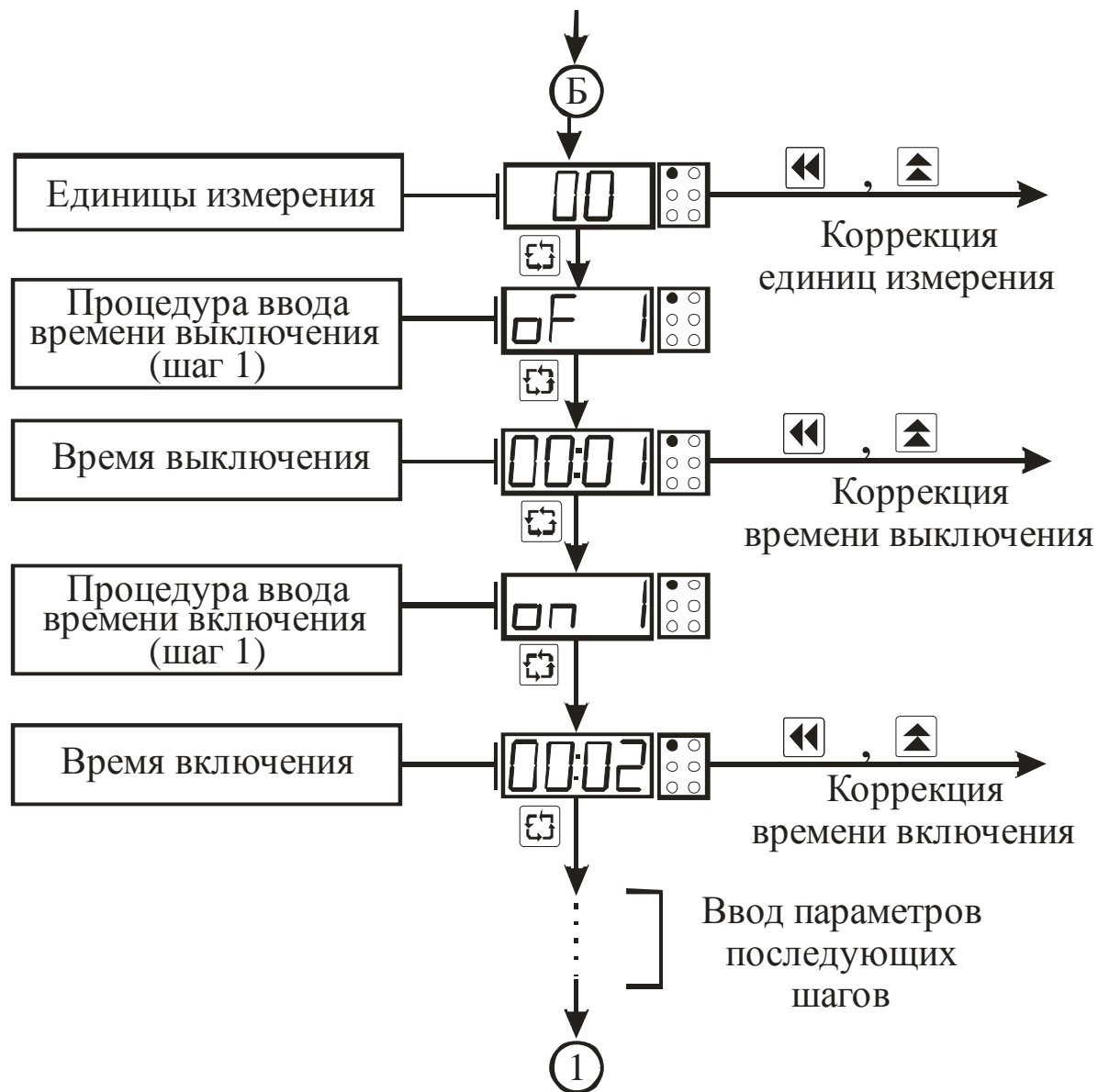
Рисунок 3.8 – Схема алгоритма работы в режиме “Параметры счёта” (продолжение)
