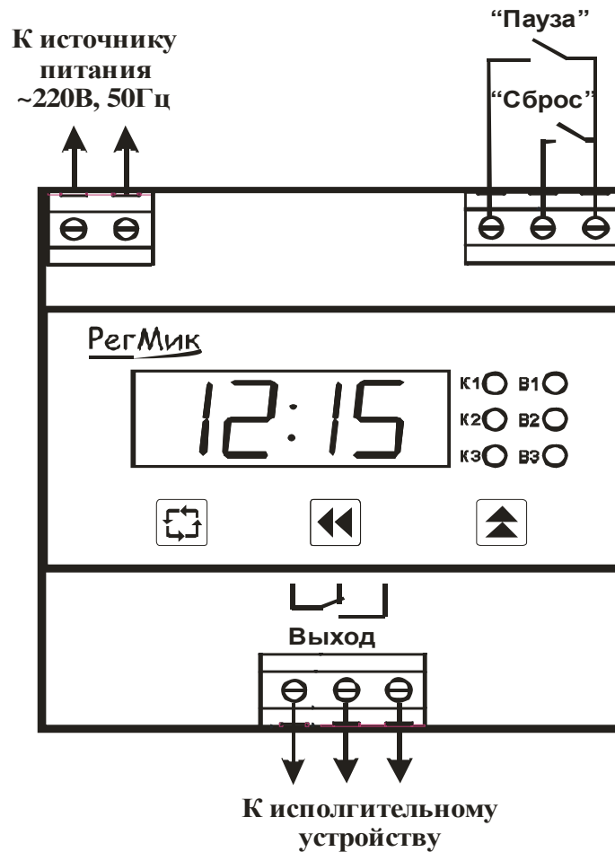
Рисунок 8.1 – Схема подключения источника питания и внешних устройств
