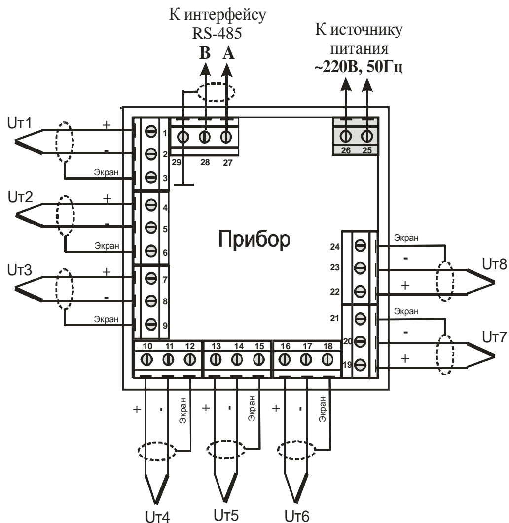
Рисунок 8.1 – Схема подключения ПТ, интерфейса связи и источника питания
