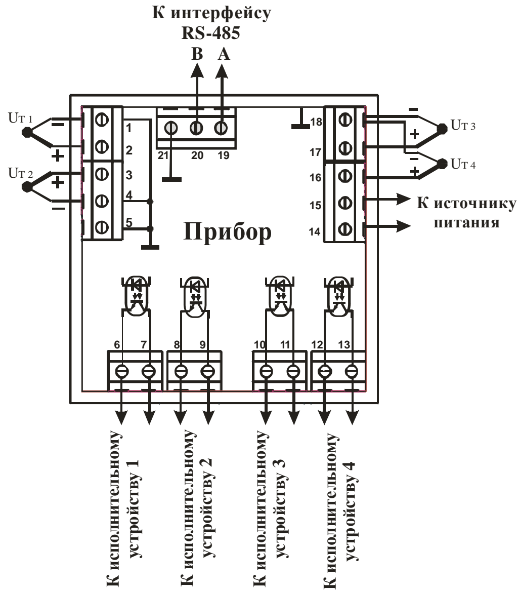
Рисунок 8.1 – Схема подключения ПТ, интерфейса RS-485, источника питания и исполнительных устройств
