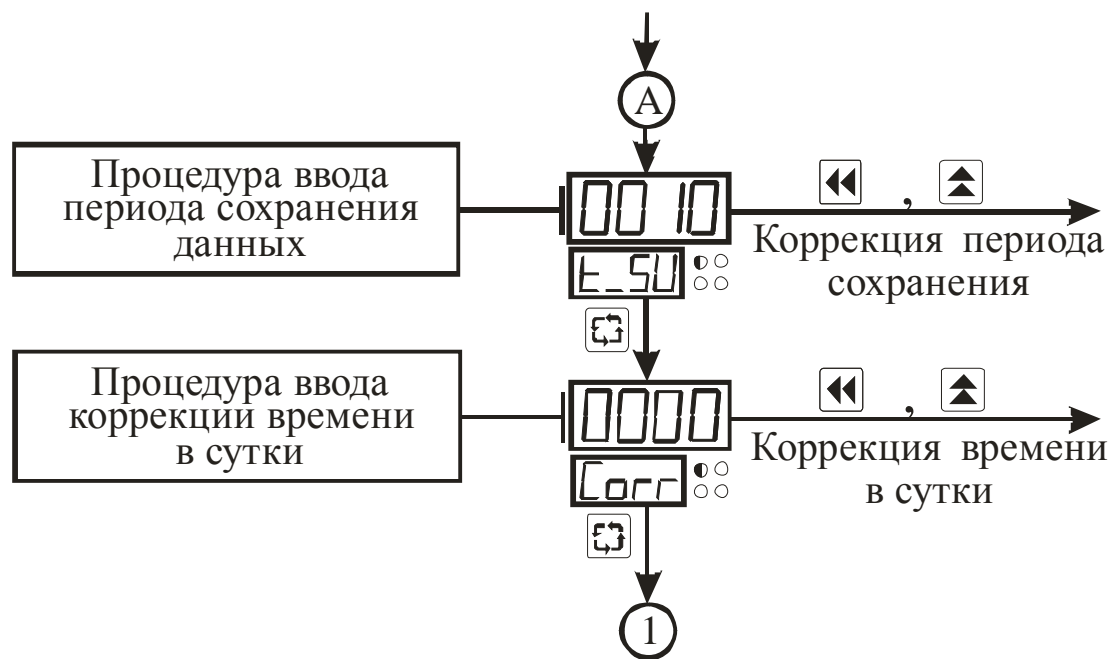
Рисунок 3.6 – Схема алгоритма работы прибора в режиме «Общие параметры» (окончание)
