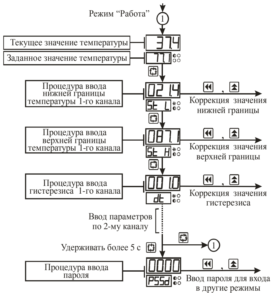
Рисунок 3.4 – Схема алгоритма работы прибора при типе логики работы выхода “03” - “05”
