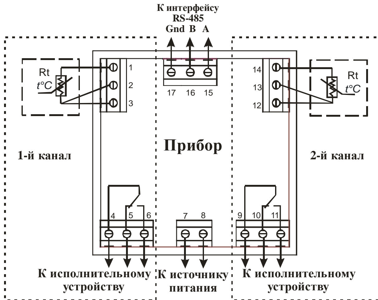
Рисунок 8.1 – Схема подключения ТС, источника питания, интерфейса RS-485 и исполнительных устройств
