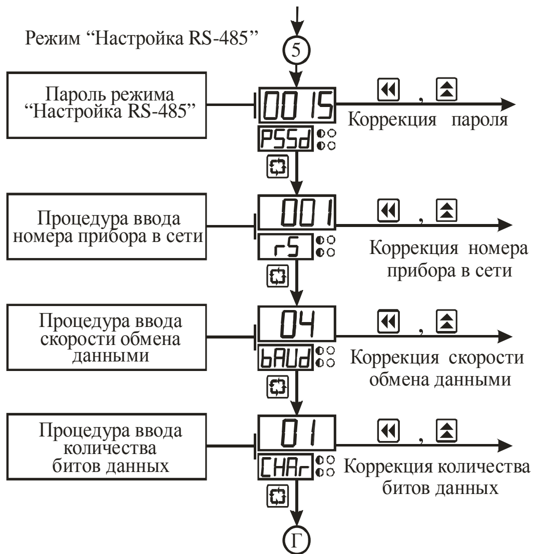
Рисунок 3.19 – Схема алгоритма работы в режиме “Настройка RS-485”
