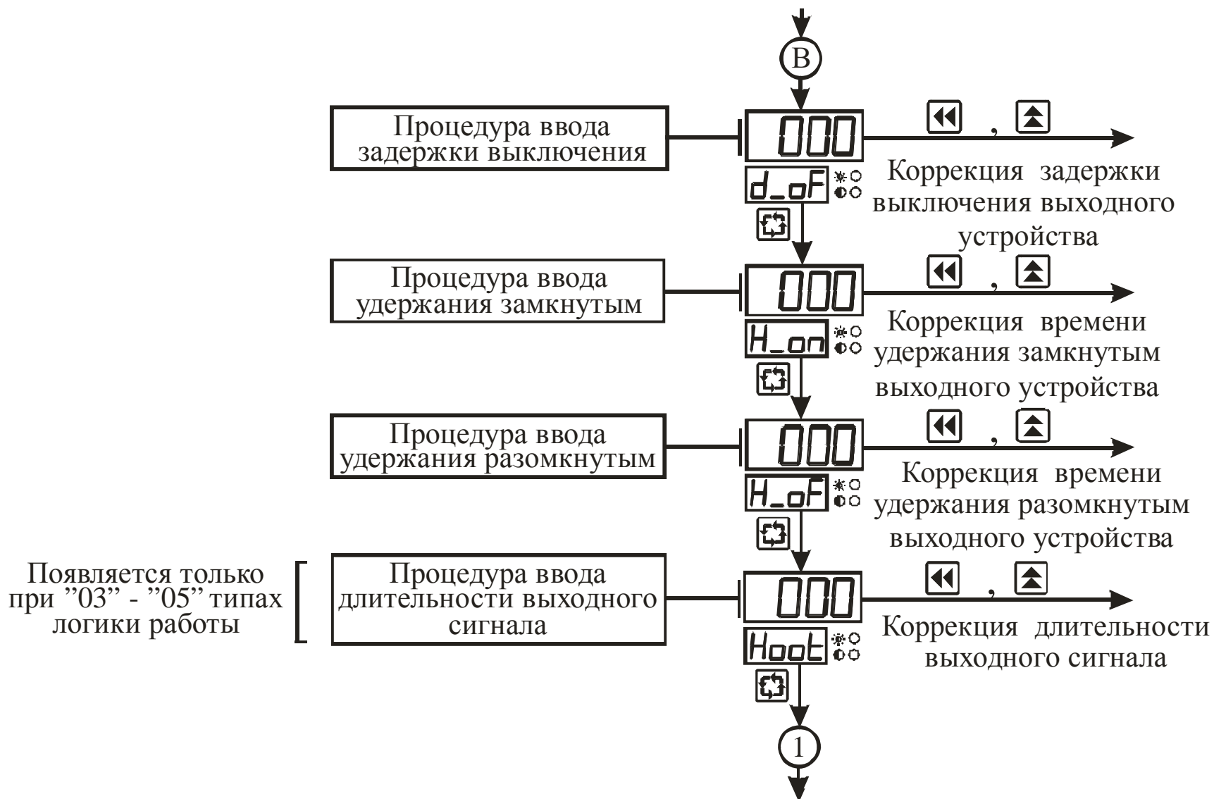
Рисунок 3.11 – Схема алгоритма работы в подрежиме “Коэффициенты 1-го канала” (окончание)
