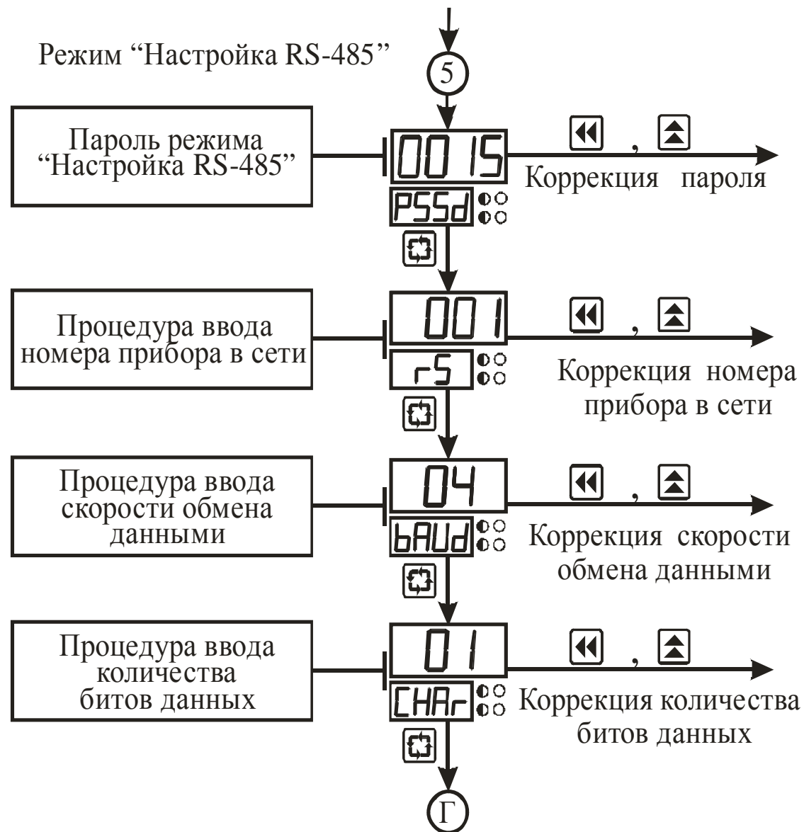
Рисунок 3.18 – Схема алгоритма работы в режиме “Настройка RS-485”
