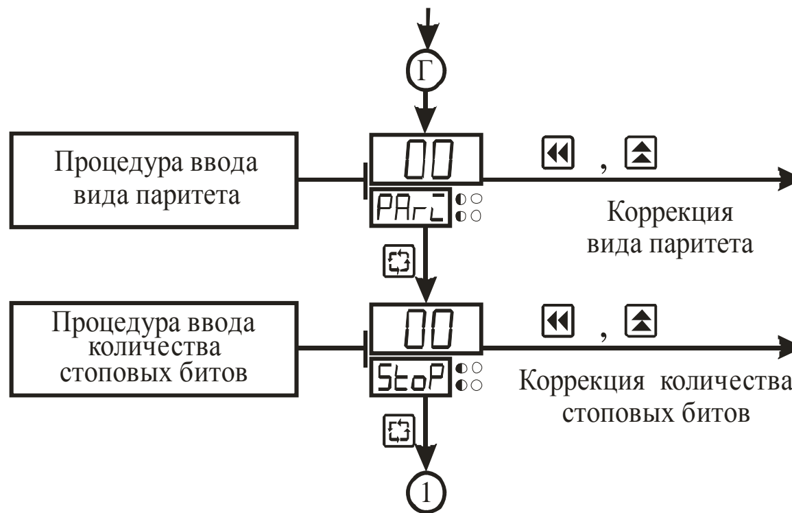
Рисунок 3.19 – Схема алгоритма работы в режиме “Настройка RS-485” (окончание)
