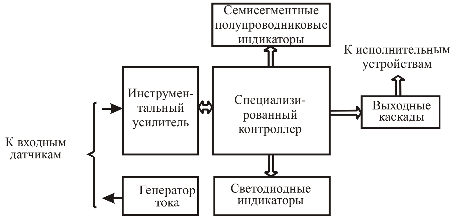
Рисунок 3.1 – Функциональная схема прибора
