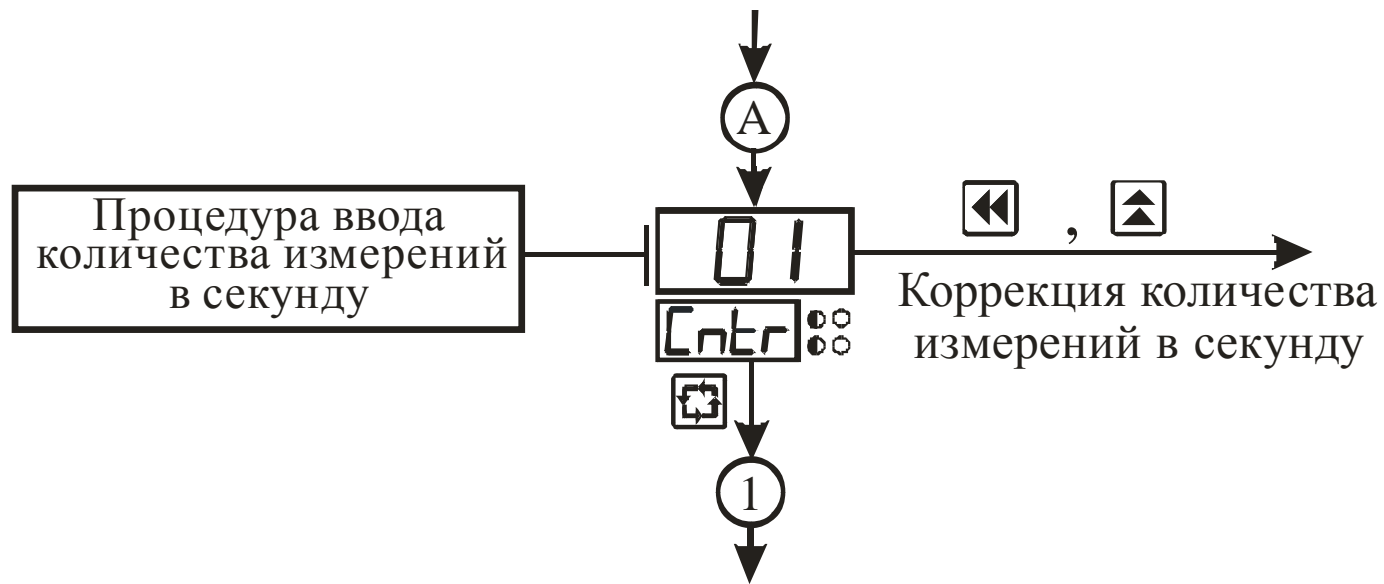
Рисунок 3.6 – Схема алгоритма работы прибора в режиме «Общие параметры» (окончание)
