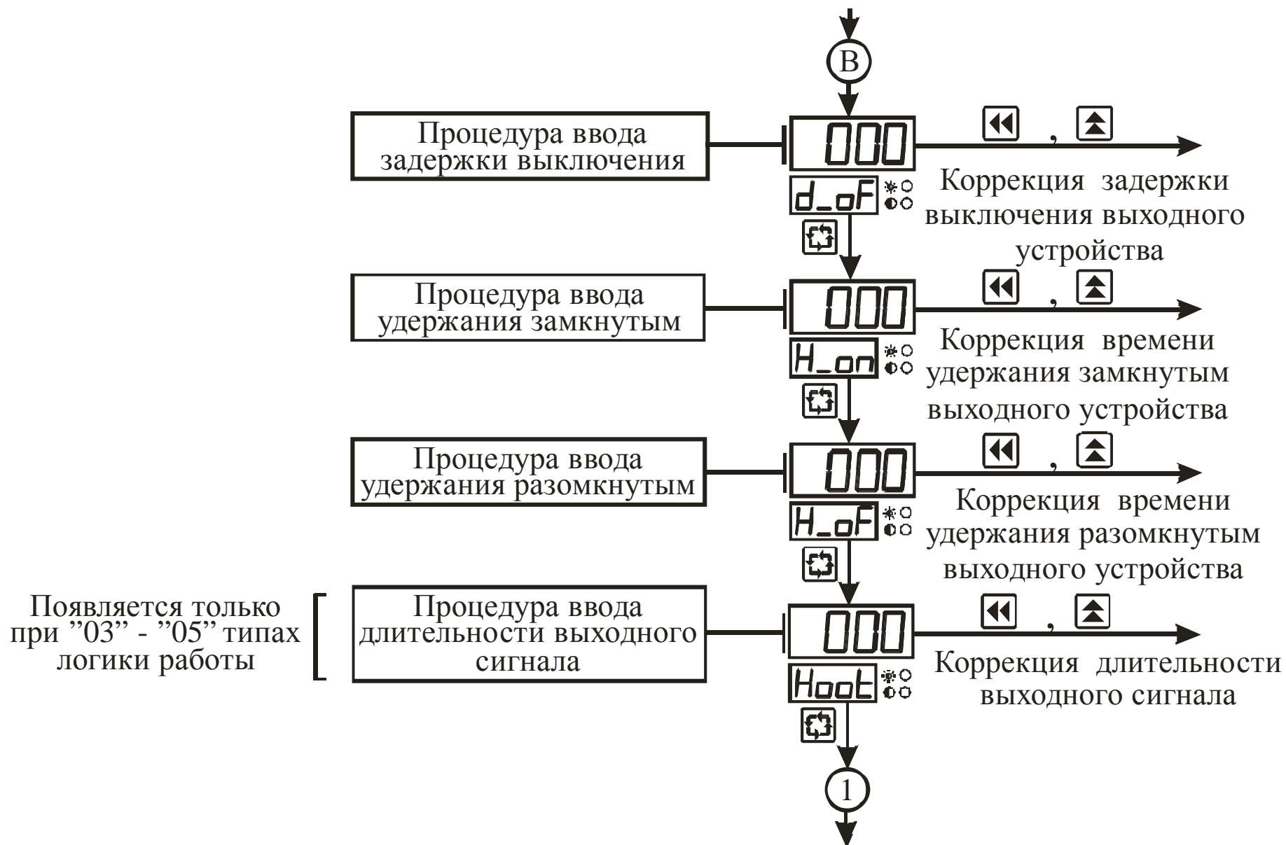
Рисунок 3.10 – Схема алгоритма работы в подрежиме “Коэффициенты 1-го канала” (окончание)
