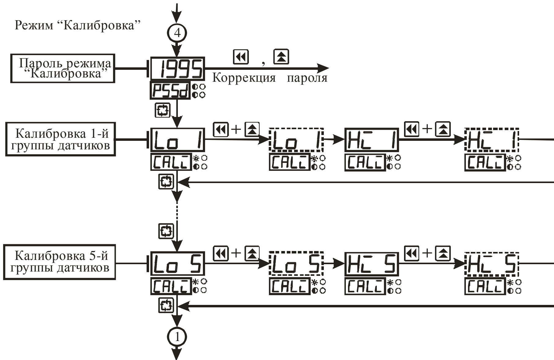
Рисунок 3.17 – Схема алгоритма работы в подрежиме “Калибровка 1-го канала”
