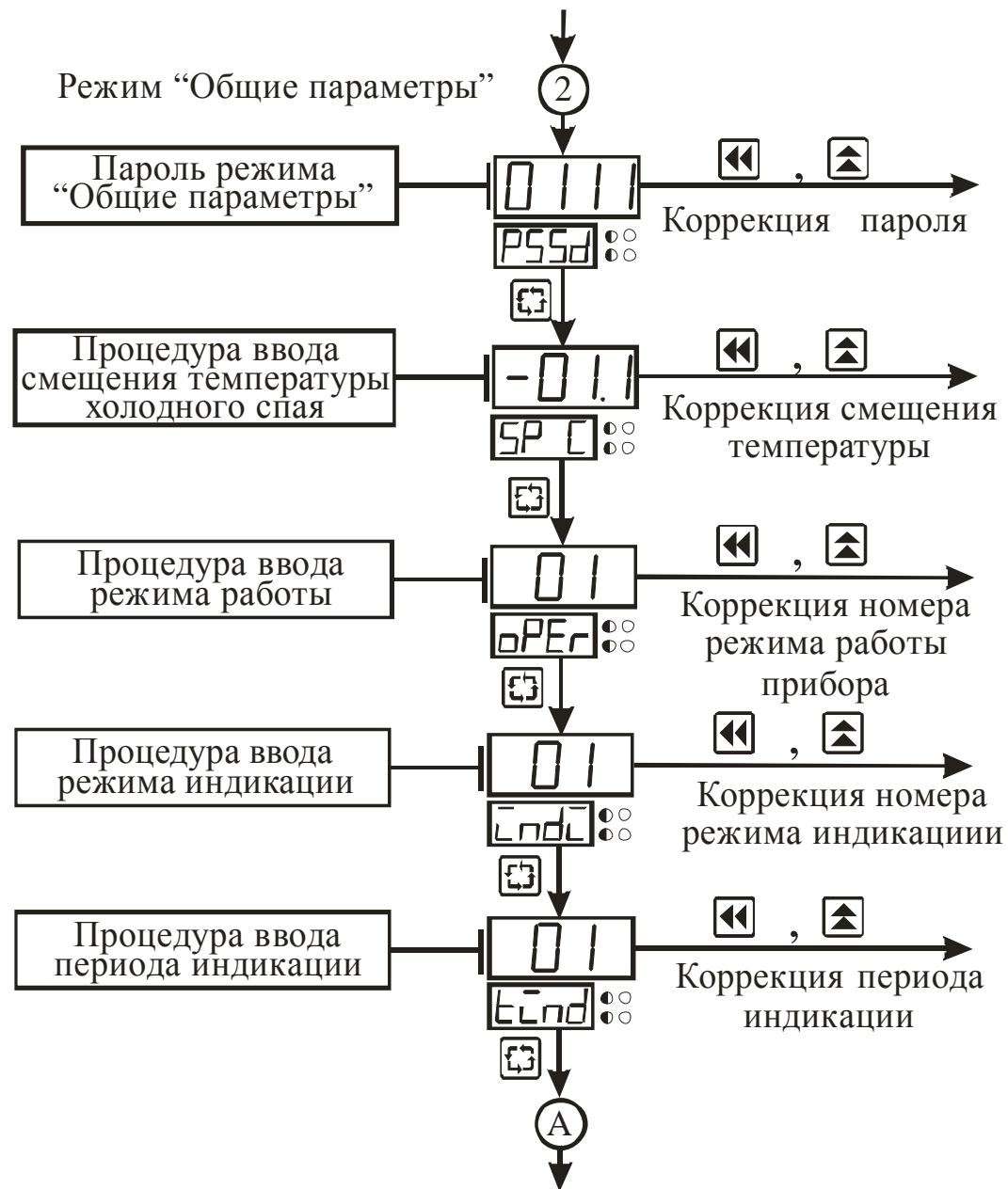
Рисунок 3.5 – Схема алгоритма работы прибора в режиме «Общие параметры»
