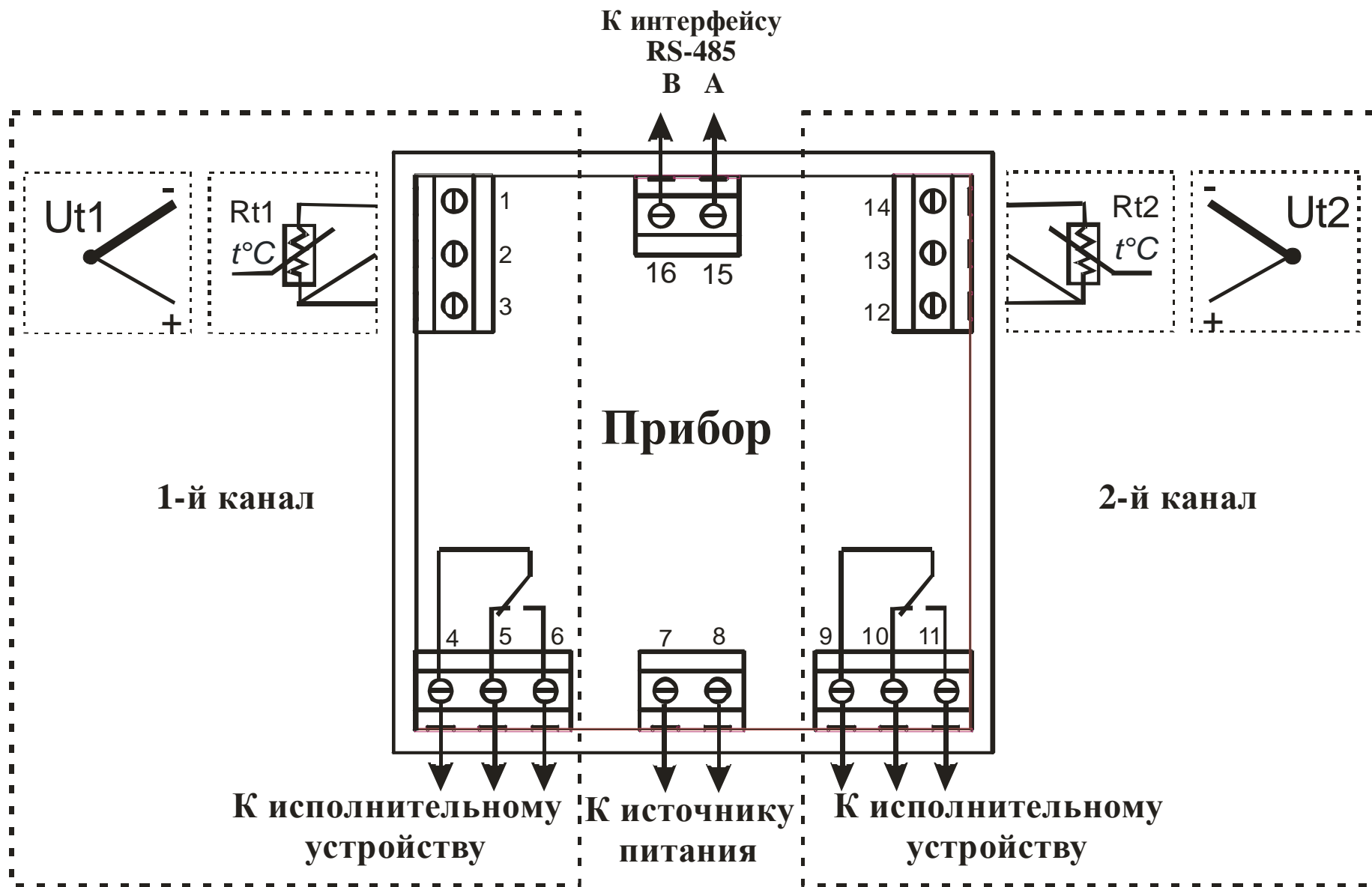
Рисунок 8.1 – Схема подключения датчиков, источника питания, интерфейса RS-485 и исполнительных устройств
