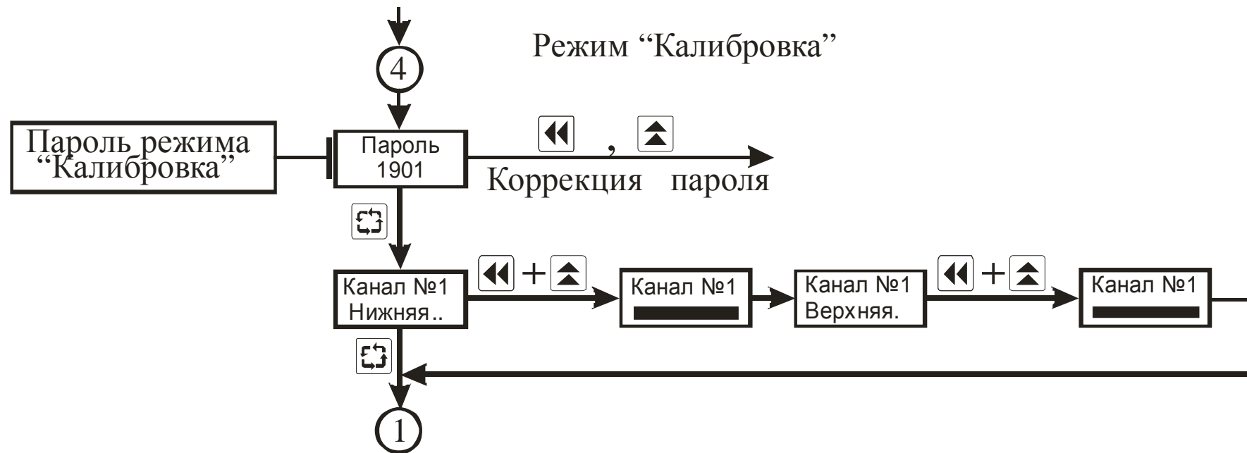
Рисунок 3.12 – Схема алгоритма работы в подрежиме “Калибровка 1-го канала”
