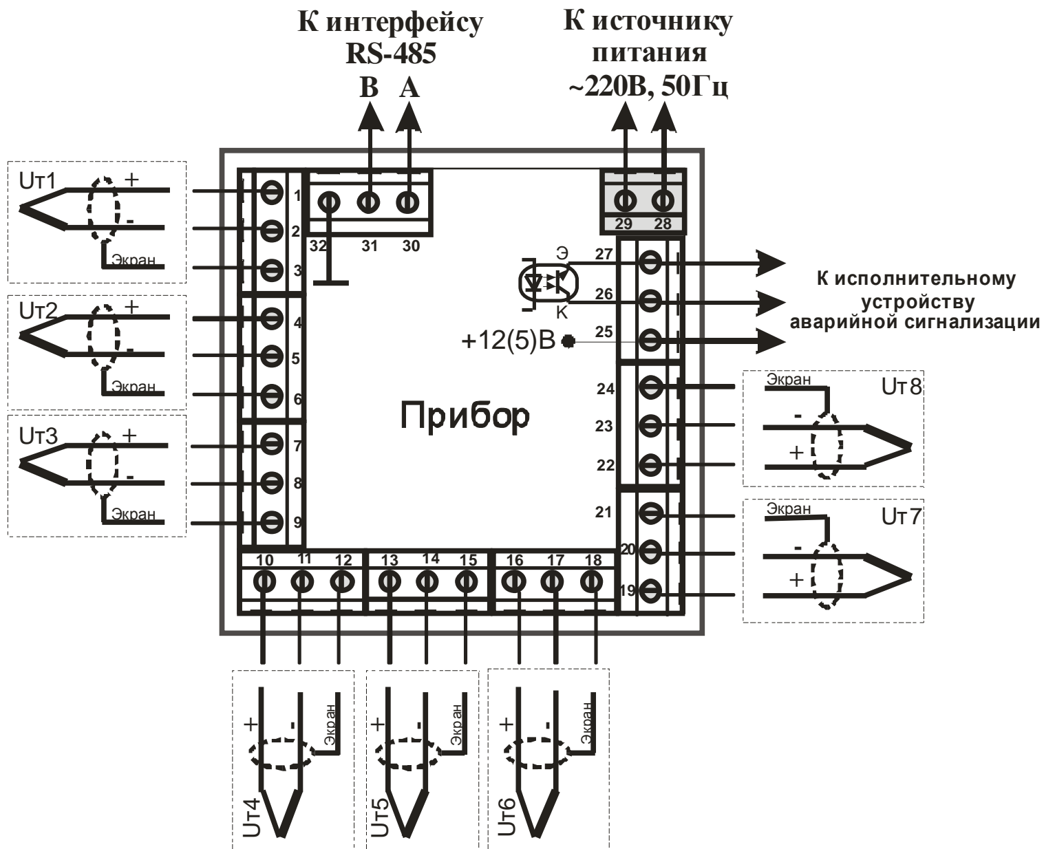
Рисунок 8.1 – Схема подключения датчиков, интерфейса RS-485 и источника питания
