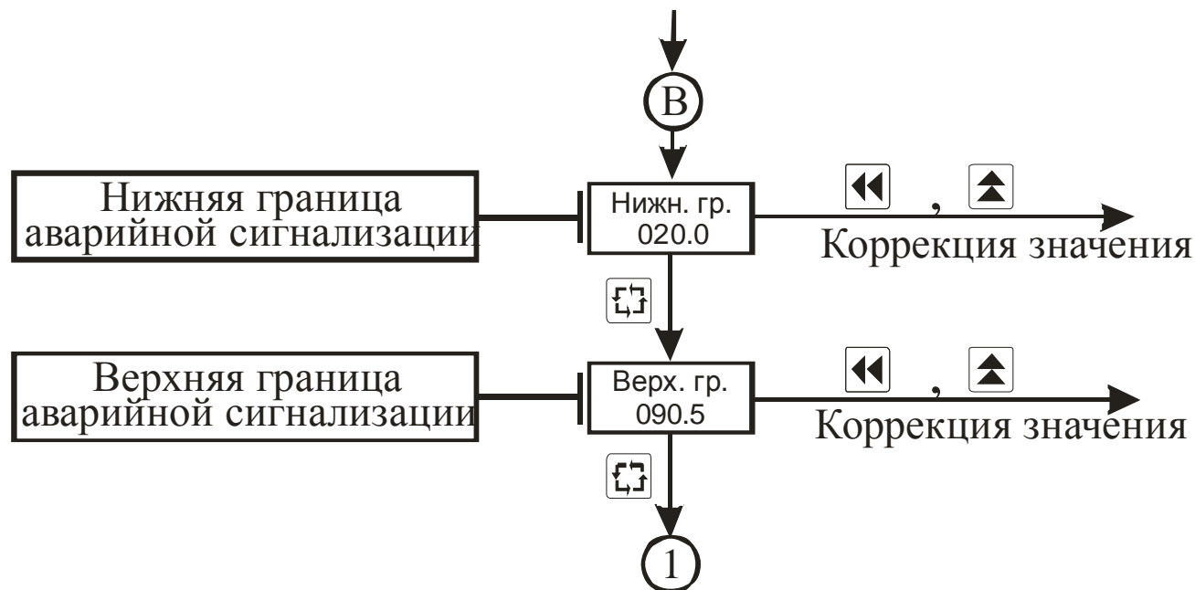
Рисунок 3.8 – Схема алгоритма работы в подрежиме “Коэффициенты 1-го канала” (окончание)
