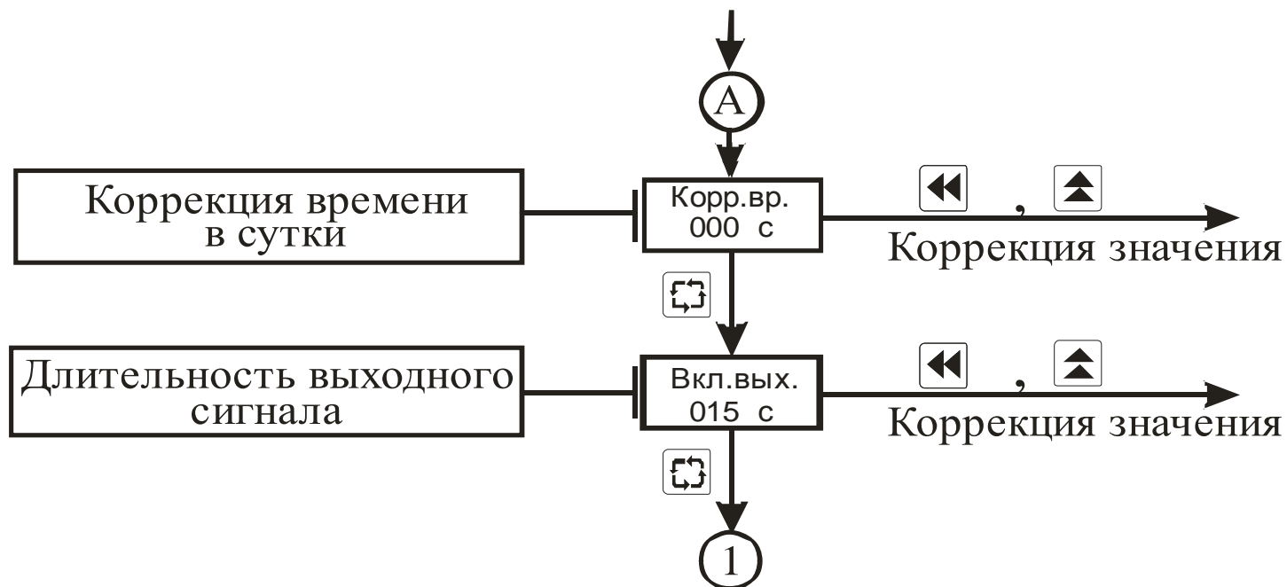
Рисунок 3.5 – Схема алгоритма работы прибора в режиме “Общие параметры” (окончание)
