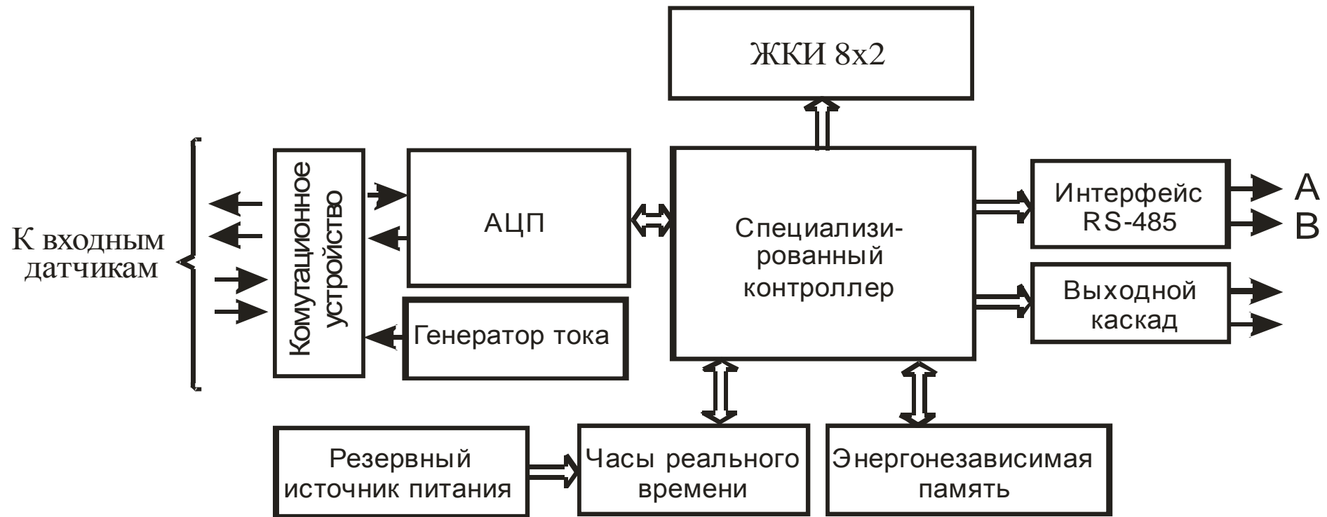
Рисунок 3.1 – Функциональная схема прибора
