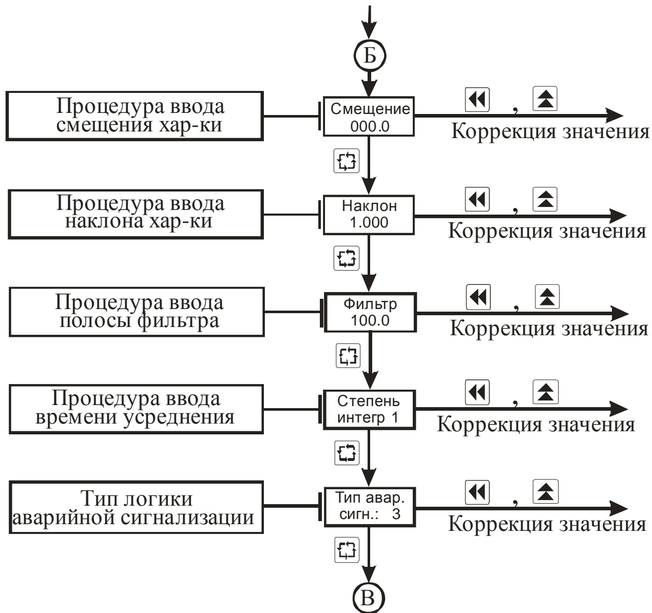
Рисунок 3.7 – Схема алгоритма работы в подрежиме “Коэффициенты 1-го канала” (продолжение)
