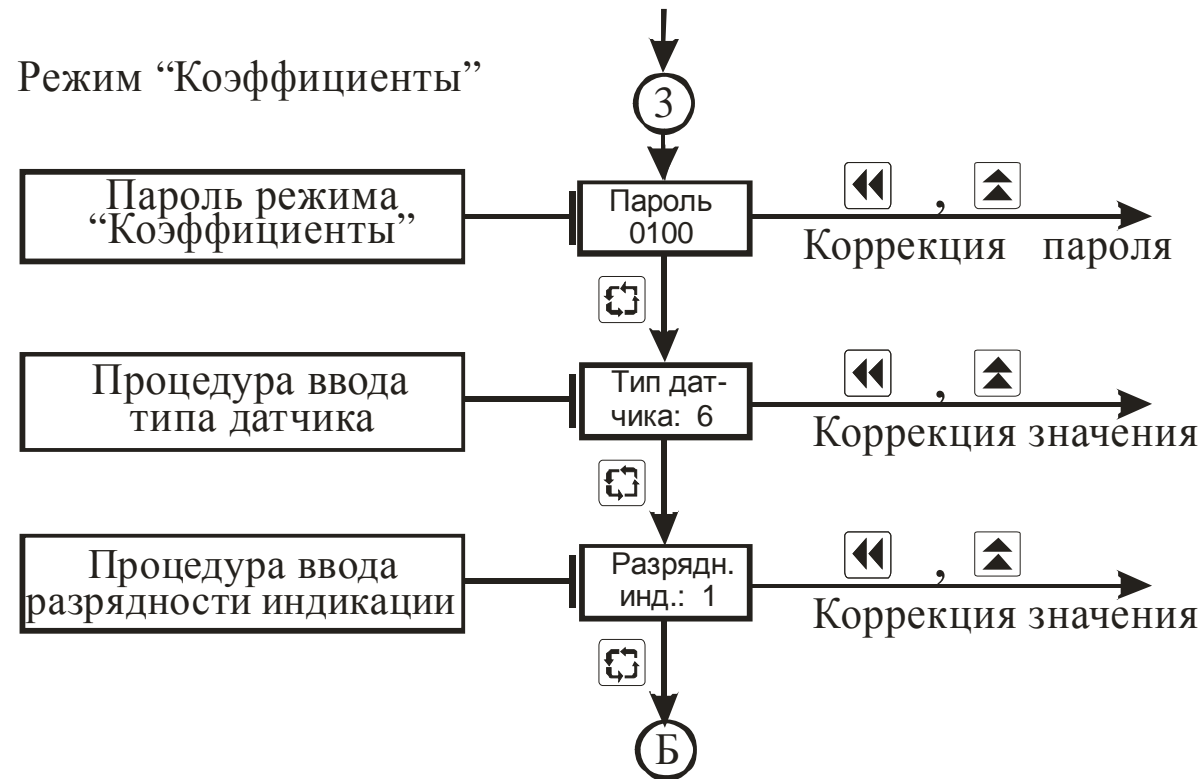
Рисунок 3.6 – Схема алгоритма работы в подрежиме “Коэффициенты 1-го канала”
