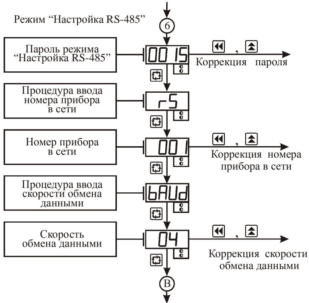
Рисунок 3.13 – Схема алгоритма работы в режиме “Настройка RS-485”
