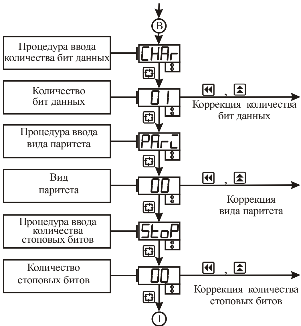
Рисунок 3.14 – Схема алгоритма работы в режиме “Настройка RS-485” (продолжение)
