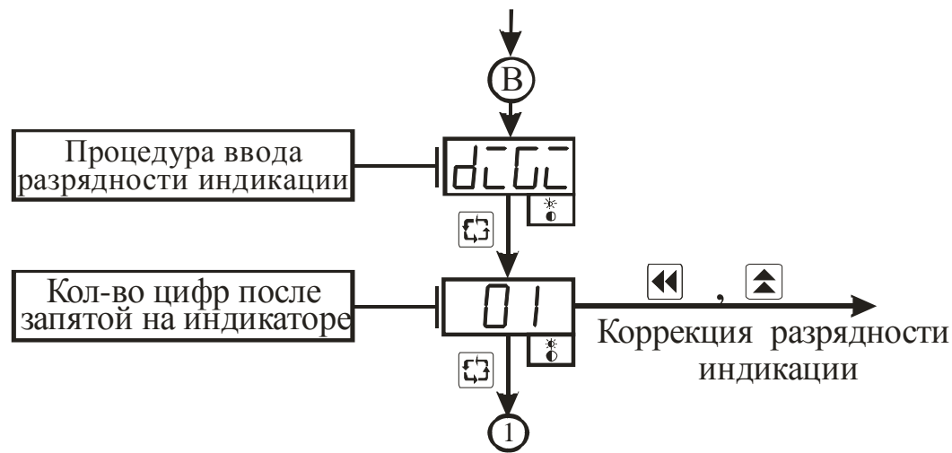
Рисунок 3.8 – Схема алгоритма работы в в подрежиме “Коэффициенты 1-го канала” (окончание)
