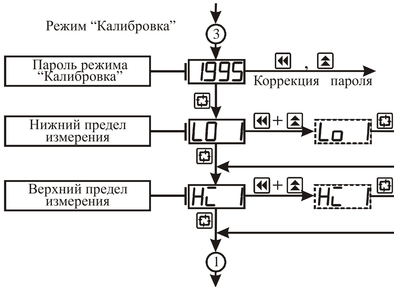
Рисунок 3.10 – Схема алгоритма работы в режиме “Калибровка”
