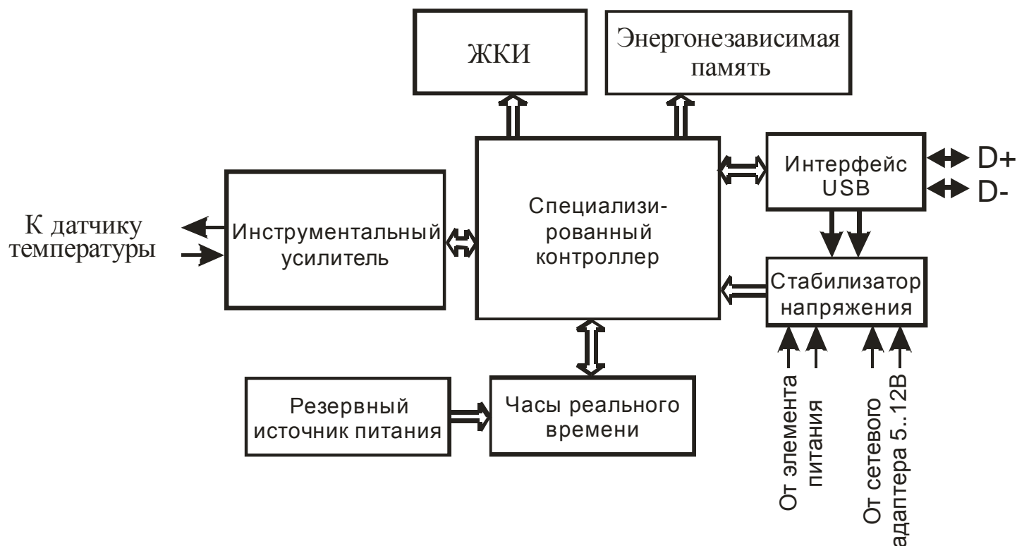
Рисунок 3.1 – Функциональная схема прибора
