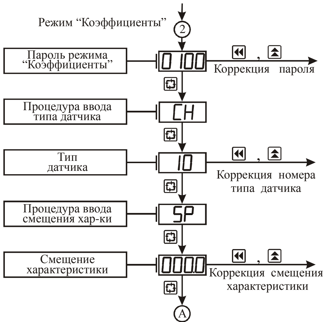
Рисунок 3.4 – Схема алгоритма работы в режиме “Коэффициенты”
