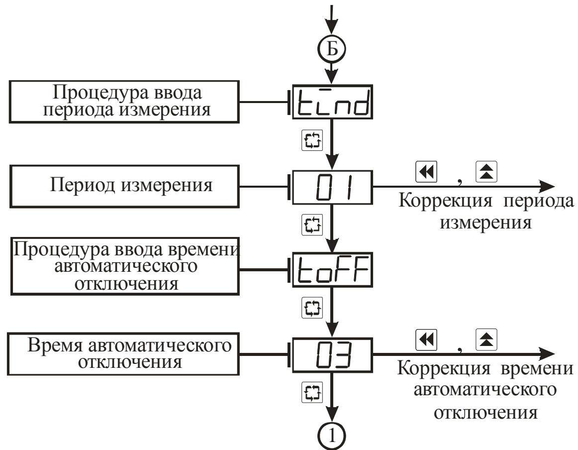
Рисунок 3.6 – Схема алгоритма работы в режиме “Коэффициенты” (окончание)
