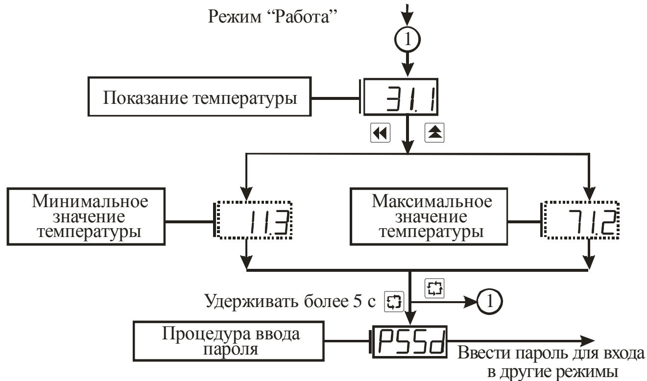
Рисунок 3.3 – Схема алгоритма работы в режиме "Работа"
