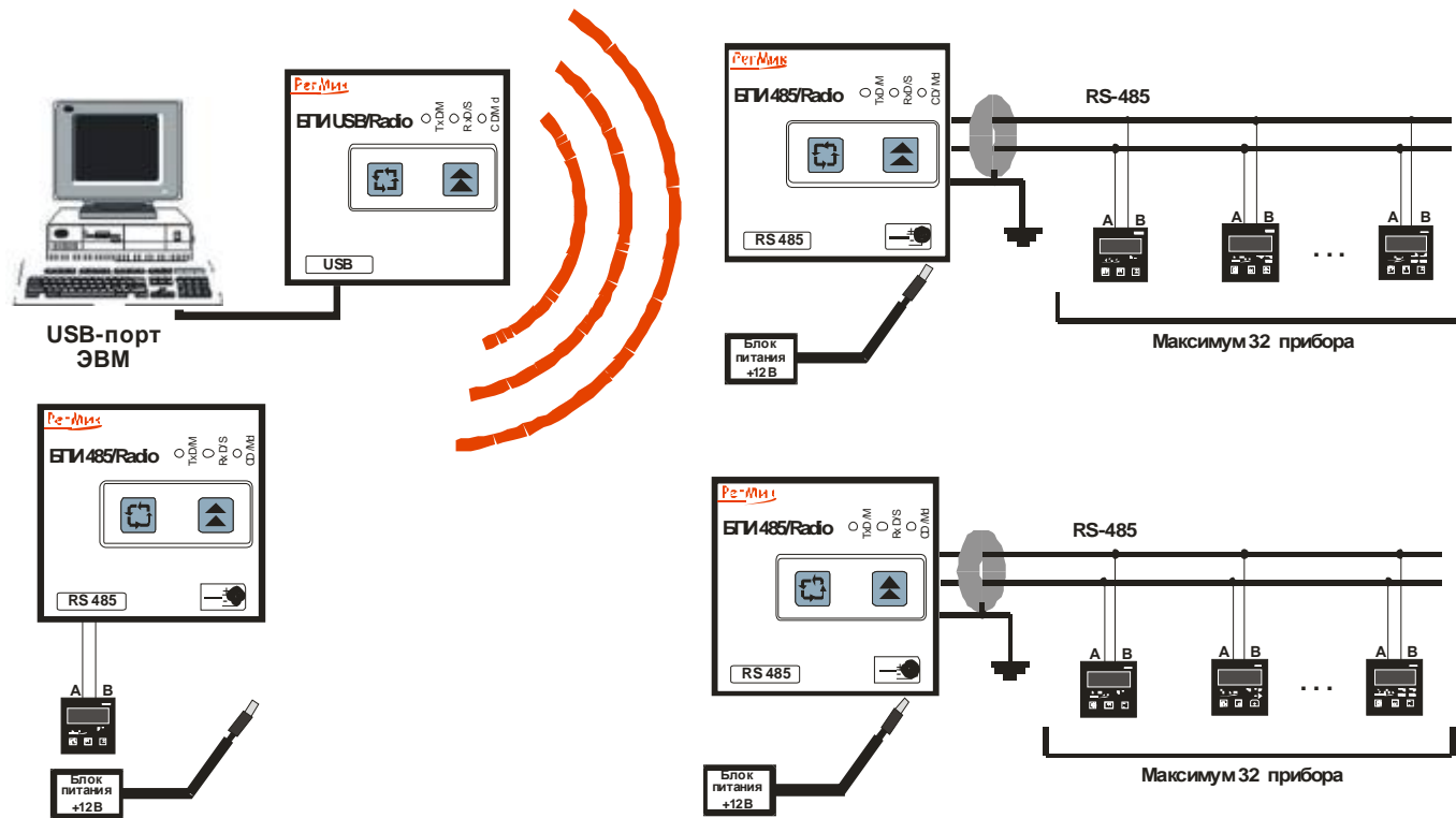
Рисунок 8.1 – Конфигурация беспроводной сети - тип звезда, (в системе ведущий и ведомые).
